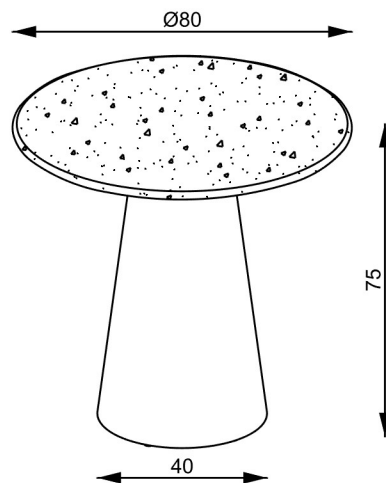
1CLSA80 - COLUNA SAVA TAMPO EM MÁRMORE Ø80 CM
