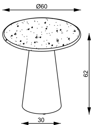
1CLSA60 - COLUNA SAVA TAMPO EM MÁRMORE Ø60 CM
